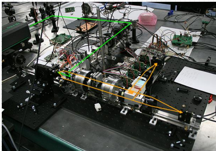
Laboratorní sestava 2016
